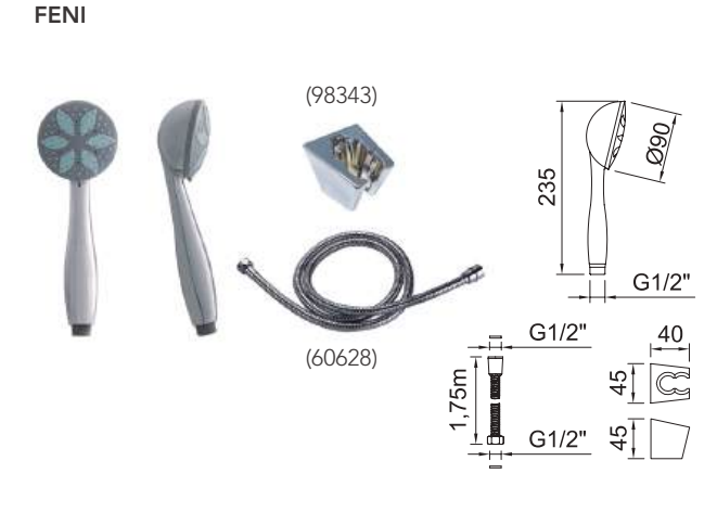
Kit de ducha Feni Ø90mm. Feni shower set Ø90mm.
