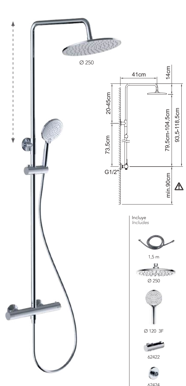
Conjunto de ducha termostática con barra extensible con soporte articulado deslizante. Thermostatic shower set with extendable bar with sliding articulated support.
