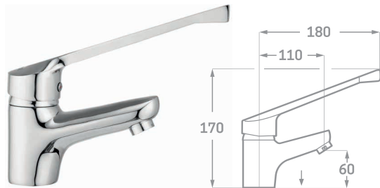
MONOMANDO LAVABO SANITARIO
