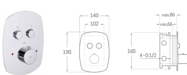
TERMOSTÁTICA DUCHA EMPOTRADA CON PULSADOR Ref. 23302RPT € 188,60
