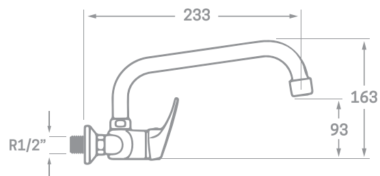
MONOMANDO FREGADERO PARED 15CM. CAÑO ALTO ACABADO CROMO
