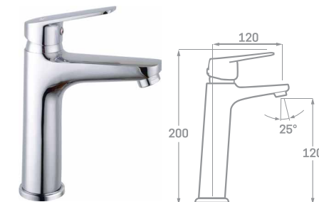
MONOMANDO LAVABO ALTO Ref. 23130A € 57,50
