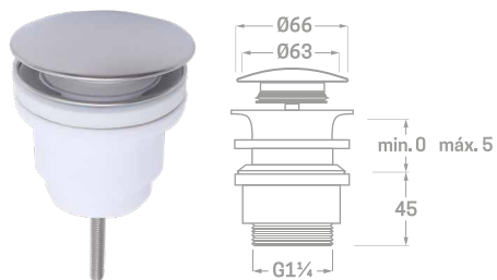
CLIC CLAC PLÁSTICO CON EJE ANTICAL BLANCO / CROMO
