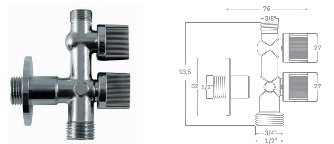
GRIFO LAVADORA ESCUADRA CON LLAVE REGULACIÓN CROMO
