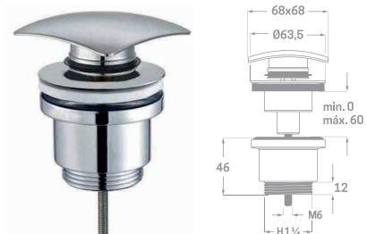
CLIC CLAC TAPÓN CUADRADO UNIVERSAL
