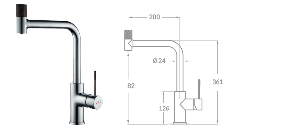
MONOMANDO FREGADERO OSMOSIS MANDO EN CAÑO ACABADO CROMO Ref. 23633 € 133,40
