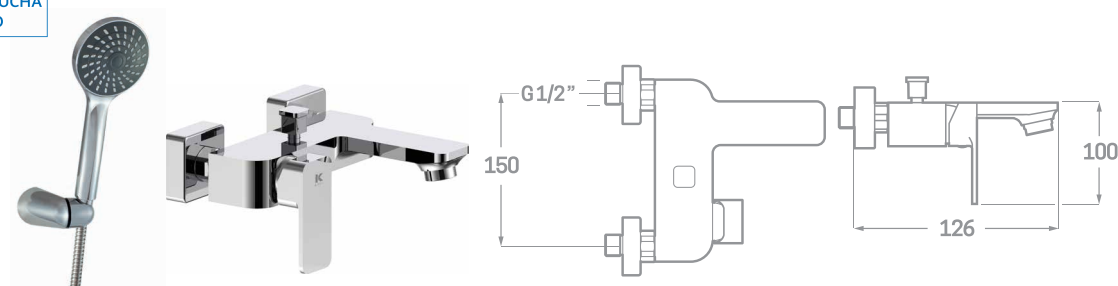
MONOMANDO BAÑO DESIGN Ref. 23419 € 131,10
