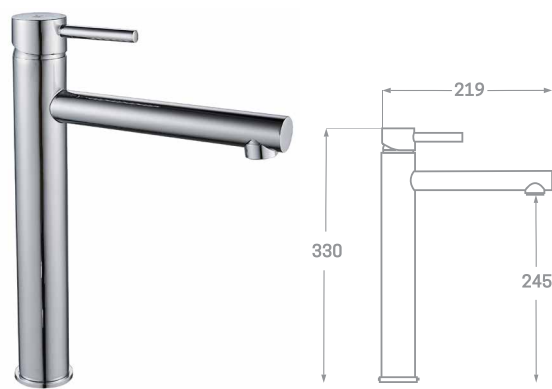
MONOMANDO LAVABO ALTO
