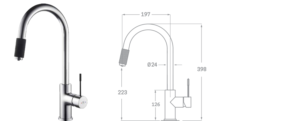
MONOMANDO FREGADERO OSMOSIS MANDO EN CAÑO CISNE ACABADO CROMO Ref. 23632 € 133,40
