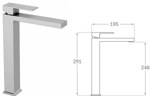
MONOMANDO LAVABO ALTO Ref. 23136A € 105,00
