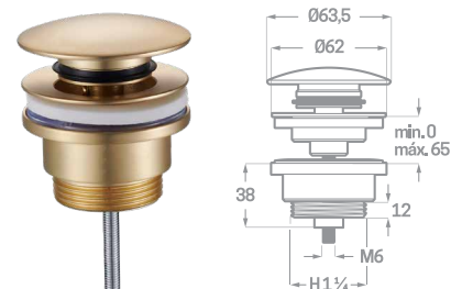
CLIC CLAC COMPACTA ORO CEPILLADO
