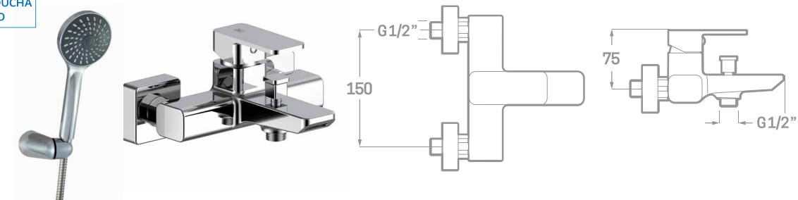
MONOMANDO BAÑO Ref. 23409 € 119,60
