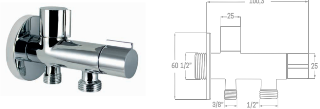
LLAVE WC CON GRIFO HIGIÉNICO 1/2 x 1/2 x 3/8 CROMO
