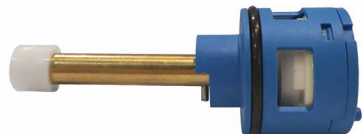
DISTRIBUIDOR CERÁMICO TIPO 12
