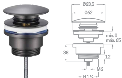
CLIC CLAC COMPACTA GRAFITO CEPILLADO
