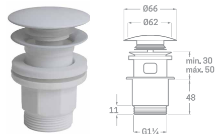
CLIC CLAC PLÁSTICO CON EJE ANTICAL TAPÓN ACERO INOX. BLANCO Ref. 06434B € 5,98
