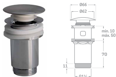
CLIC CLAC PLÁSTICO CON EJE ANTICAL LARGA TAPÓN ACERO INOX. PULIDO Ref. 06435 € 6,33
