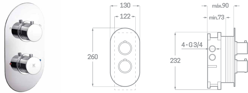
TERMOSTÁTICA DUCHA EMPOTRADA DESIGN Ref. 23302RTV € 200,10
