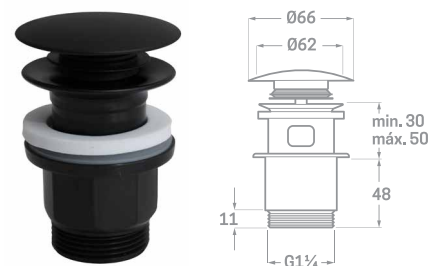
CLIC CLAC PLÁSTICO CON EJE ANTICAL TAPÓN ACERO INOX. NEGRO MATE Ref. 06434N € 6,14
