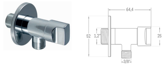
LLAVE ESCUADRA NOVA 1/2 x 3/8 CROMO
